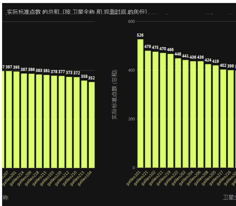
1.6.3 GALILEO
