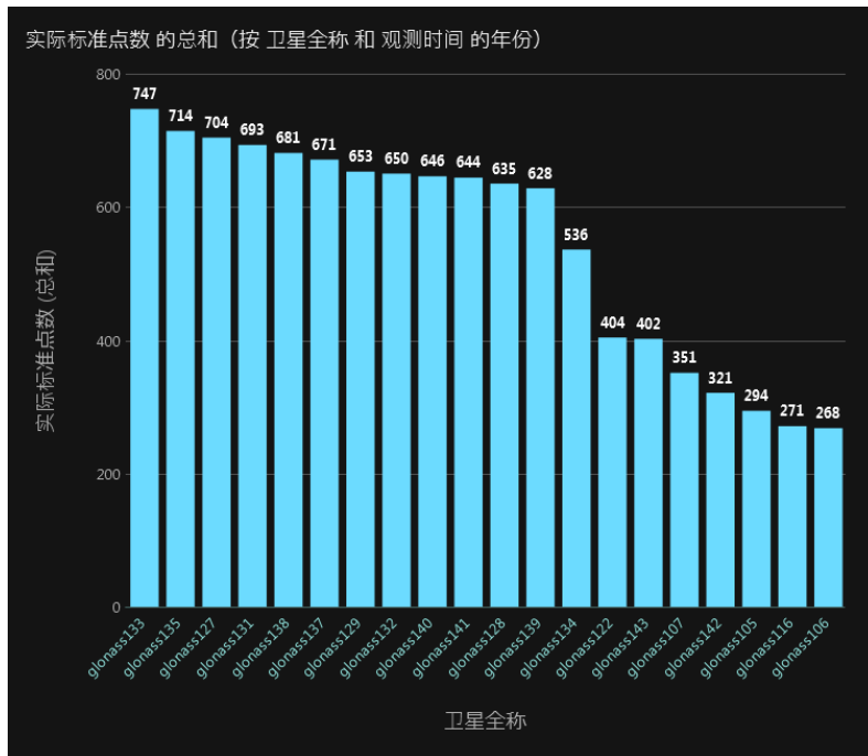
1.6.2 GLONASS
